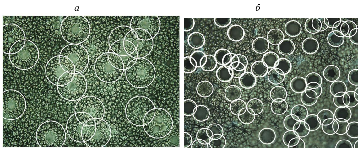
Рис. 3. Определение кластеров на поверхности электролитических никелевых пен. Время получения пен электролизом, мин: а – 5, б – 25.
