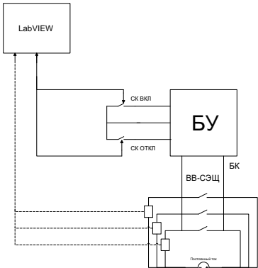
Рис. 1. Схема лабораторного стенда (шрифт 11, по центру) [источник их списка литературы]
